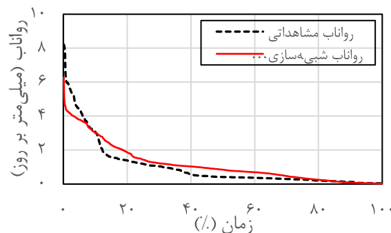
شکل ۱۶- منحنی تداوم رواناب مشاهداتی و شبیه‌سازی شده مدل هیدرولوژیکی SimHyd برای مرحله صحت‌سنجی
