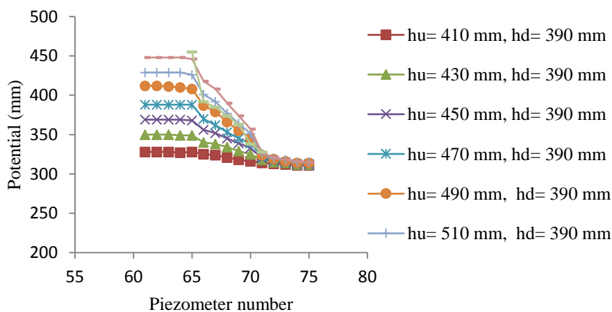
شکل ۳- تغییرات پتانسیل برای پی با D_{50}=0.2\text{ mm} و h_d=390\text{ mm}
