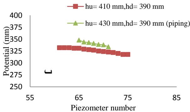
شکل ۱۱- تغییرات پتانسیل الف- آرایش سه لایه ۰/۲-۱/۲-۰/۶ میلیمتر، بدون پرده آب‌بندب- آرایش سه لایه ۰/۲-۰/۶-۱/۲ بدون پرده آب‌بند
