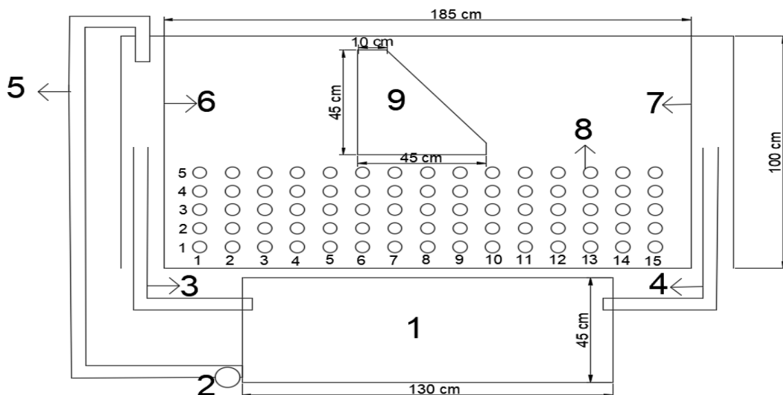
شکل ۱- تصویر شماتیک مدل آزمایشگاهی و محل قرارگیری پی‌زومترها
