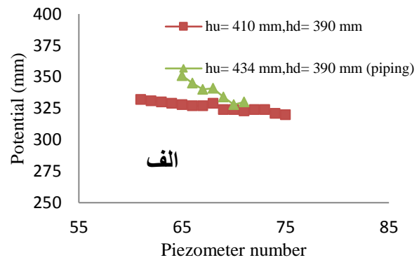
شکل ۱۲- تغییرات پتانسیل الف- آرایش سه لایه ۰/۲-۱/۲-۰/۶ میلیمتر، بدون پرده آب‌بندب- آرایش سه لایه ۰/۲-۰/۶-۱/۲ بدون پرده آب‌بند
