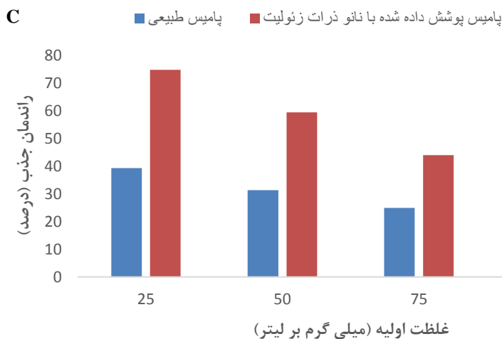
شکل ۶. نمودار اثر زمان تماس بر روی راندمان حذف نیترات توسط سنگدانه های پامیس طبیعی و اصلاح شده در شرایط بهینه (A)، تاثیر مقدار غلظت‌های اولیه متفاوت بر ظرفیت جذب نیترات در شرایط بهینه (B) و تاثیر مقدار غلظت‌های اولیه متفاوت بر راندمان حذف نیترات در شرایط بهینه (C)
