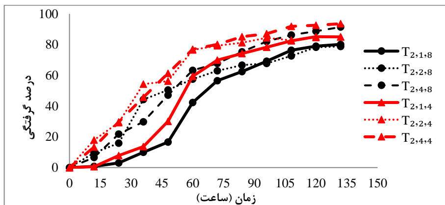
شکل ۷- روند تغییرات گرفتگی قطره‌چکان‌های با فشار کارکرد ۲/۱۰ بار، تحت انقطاع‌های یک، دو و چهار بار در هر ۴ ساعت کارکرد
