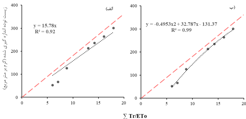
شکل ۳-الف- مقایسه ضریب WP^* در کشت اول برای تیمار N0 توسط رگرسیون خطی (ب) توسط رگرسیون غیرخطی (خط قرمز رنگ معرف شاخص WP^* در حالت پتانسیل و بدون تنش حاصلخیزی است ( y=18.1x ))
