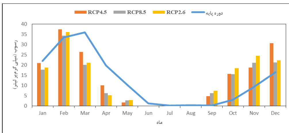
شکل ۸- میانگین رسوب ماهانه دوره پایه و دوره آتی
