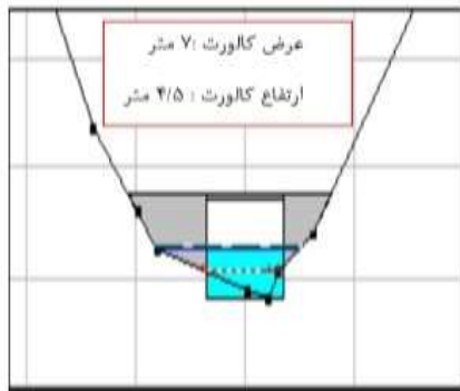
شکل ۵- کانال سرپوشیده در بالادست منطقه امامزاده داوود
