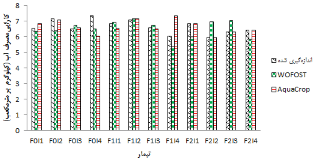
شکل ۳- نتایج بهره‌وری آب مشاهداتی چغندر نسبت به مقادیر شبیه‌سازی شده با مدل‌های AquaCrop و WOFOST
