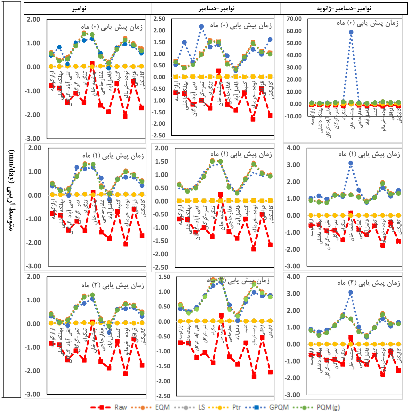
شکل ۲- متوسط اریبی پیش‌بینی‌های خام و تصحیح شده (mm/day)
