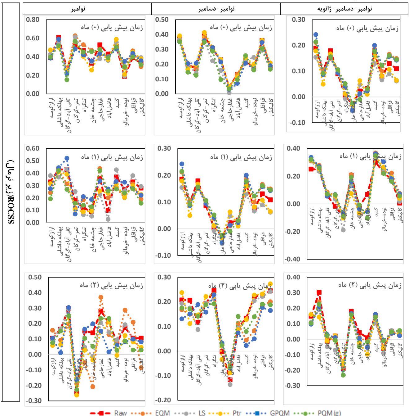
شکل ۴ - ROCSS برای شرایط زیر نرمال قبل و بعد از اعمال روش‌های تصحیح اربینی
