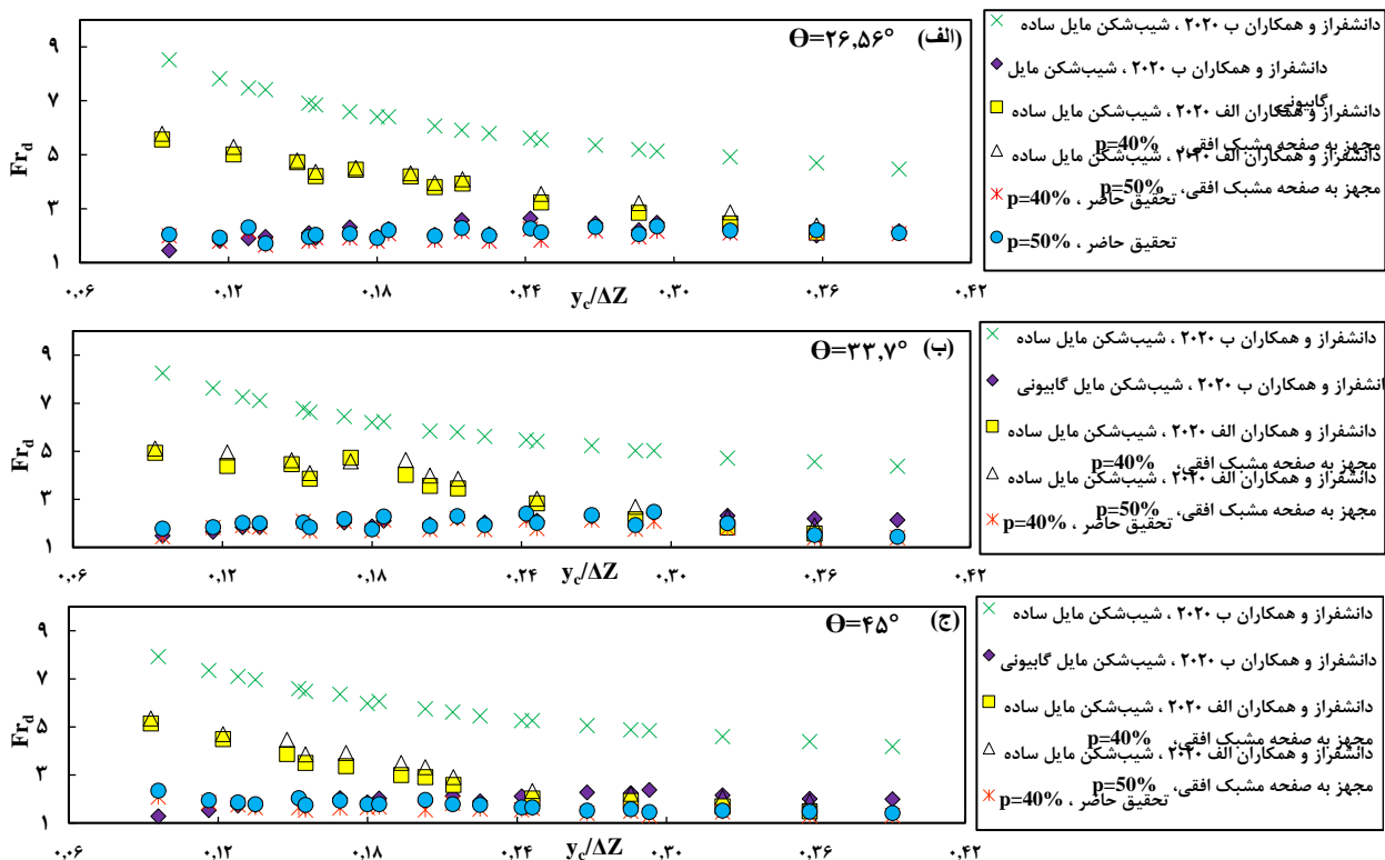
شکل ۸- تغییرات عدد فرود پایین‌دست در مقابل عمق بحرانی نسبی
