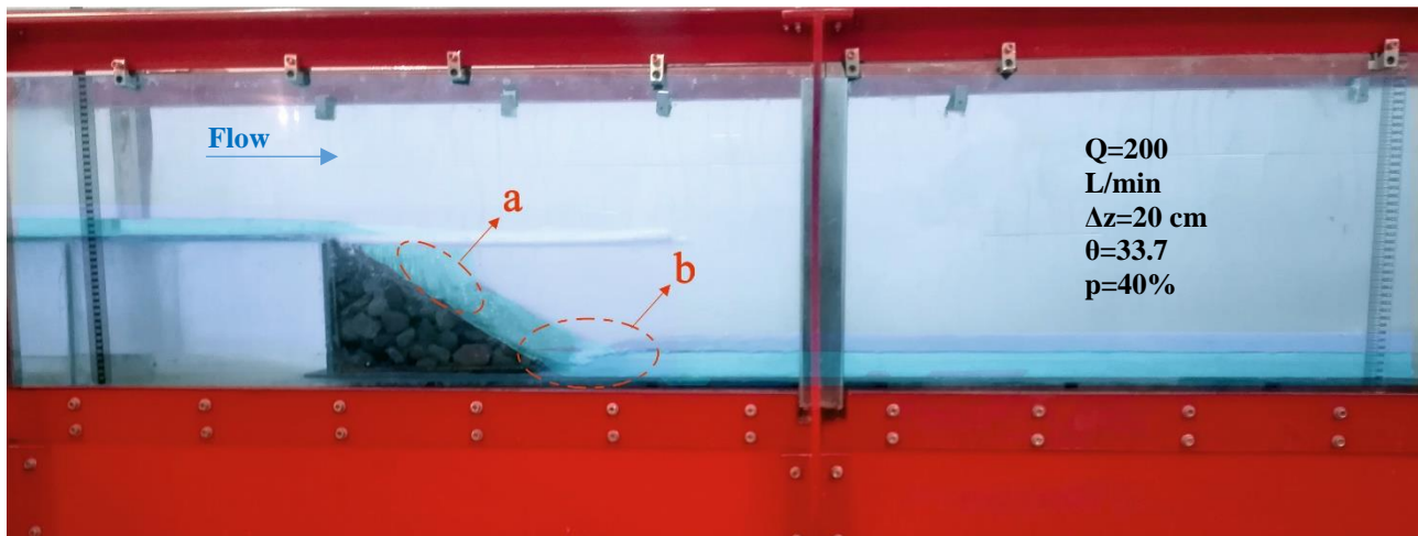
شکل ۳- نمایی از جریان در حالت درون‌گذر
