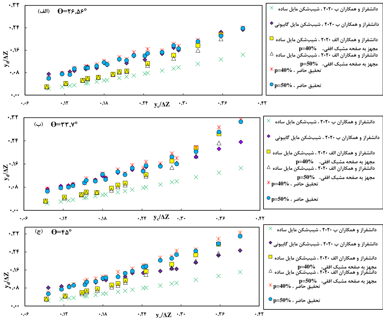
شکل ۷- تغییرات عمق نسبی پایین دست در مقابل عمق بحرانی نسبی
