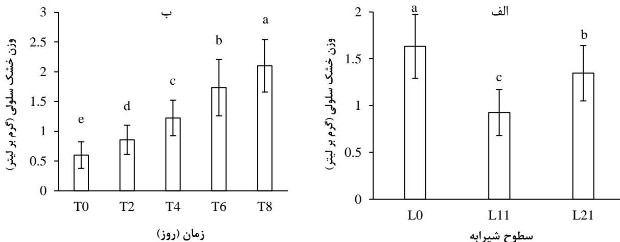
شکل ۱- پیامد سطوح شیرابه (الف) و زمان (ب) بر وزن خشک یاخته در ریزجلبک کلرلا ولگاریس. بودن حداقل یک حرف مشترک روی ستون‌ها نشان دهنده نبودن تفاوت آماری معنی دار در سطح احتمال ۵ درصد است. نوارهای خطا نشان دهنده انحراف از معیار هستند. مقادیر میانگین ۳ تکرار هستند. بدون شیرابه (L0)، شیرابه با رقت ۱:۱ (L11) و شیرابه با رقت ۲:۱ (L21)
