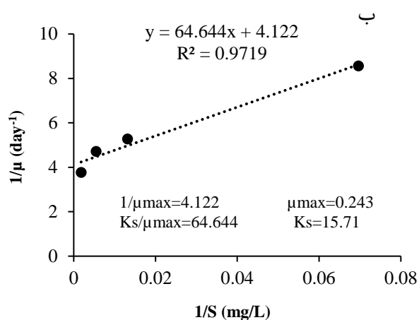
شکل ۷- تعیین بیشینه سرعت رشد ویژه ( \text{day}^{-1} ) و ضرب مونود ( \text{mg L}^{-1} ) فسفات و (ب) آمونیوم با بهره‌گیری از طرح لینیویر-برک بر اساس ترسیم 1/\mu در مقابل 1/S
