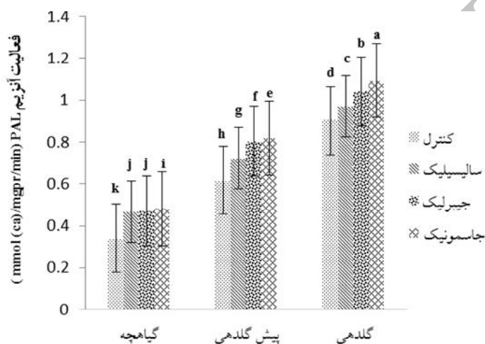
شکل ۴- میزان فعالیت آنزیم فنیل آلانین آمونیا لیااز در برگ‌های ریحان با تیمار متقابل تنظیم‌کننده‌های رشد و مراحل رشد گیاهی. حروف متفاوت بالای نمودارها نشان‌دهنده معنی‌دار بودن در سطح ( P \leq 0.05 ) می‌باشد.
