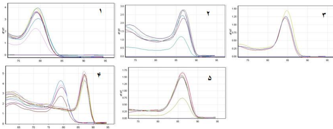
شکل ۲. منحنی ذوب ژن‌های مورد مطالعه با استفاده از تکنیک QRT-PCR. ۱- ژن CYP81Q1 ، ۲- ژن CYP81Q2 ، ۳- ژن 18S ، ۴- ژن rRNA و ۵- ژن CYP81Q3 و C3H .
