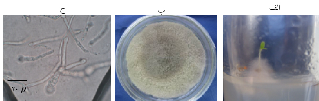
شکل ۵- Penicillium implicatum جدا سازی شده از بذر توس (الف) پرگنه بر روی PDA، (ب و ج) کنیدیفور و کنیدی‌ها
