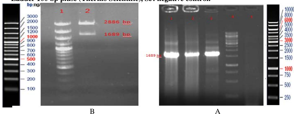
شکل ۲- A- الگوی الکتروفورزی ژل آگارز (یک درصد) واکنش کلونی PCR، ستون ۱ و ۲ و ۳ کلونی PCR، ستون ۴ نشانگر 1kb (Thermo Scientific) 1kb- B. ستون ۱- نشانگر 100 bp (Thermo Scientific) pluse و ستون ۲: هضم دو آنزیمی pTZ57R/TP1- InvG .
