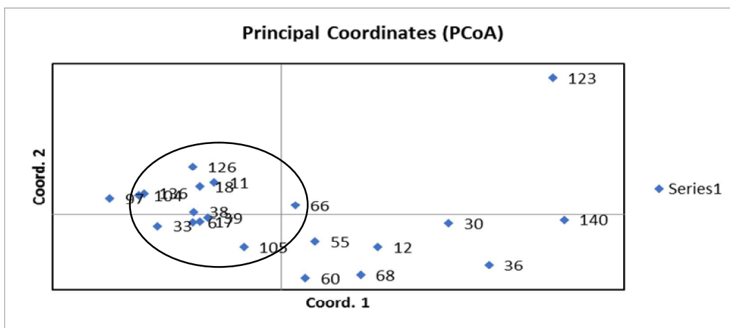
شکل 1. نمایش دو بعدی تجزیه مؤلفه اصلی بر اساس مؤلفه اول و دوم داده‌های نشانگر AFLP
