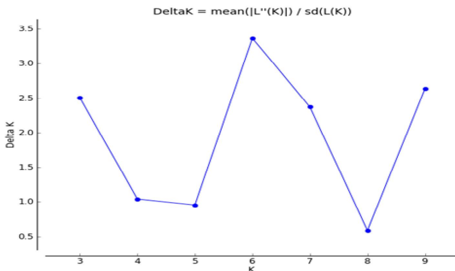
شکل 2. نمودار نتایج روش اوانو در انتخاب K بهینه
