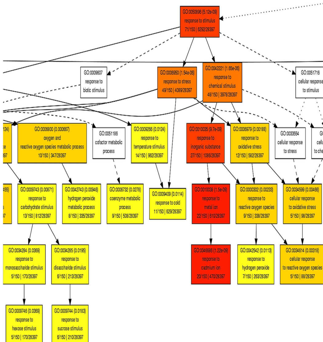
شکل ۳. نمودار درختی فرآیندهای زیستی غنی شده مرتبط با ۱۵۰ پروتئین ناپدید شده به دنبال از کار انداختن ژن AT2G37050 . این شکل با الگوریتم agriGO و با روش SEA ترسیم شده است. در هر مربع فرآیند زیستی به همراه کد GO term و اطلاعات آماری قید شده است. GO term معنی دار ( P \leq 0.05 ) با رنگ نمایش داده شده است و مربع‌های سفید رنگ GO term که از لحاظ آماری بی معنی است را نشان می‌دهد. شدت رنگ هر مربع با درجه غنی‌شدگی فریند زیستی ارتباط مستقیم دارد. تصویر کامل این نمودار درختی در شکل تکمیلی SF1 نمایش داده شده است.
