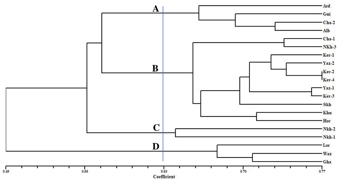
شکل ۲. تجزیه خوشه‌ای ژنوتیپ‌های بونه وحشی به روش UPGMA براساس داده‌های مولکولی حاصل از تجزیه ISSR
