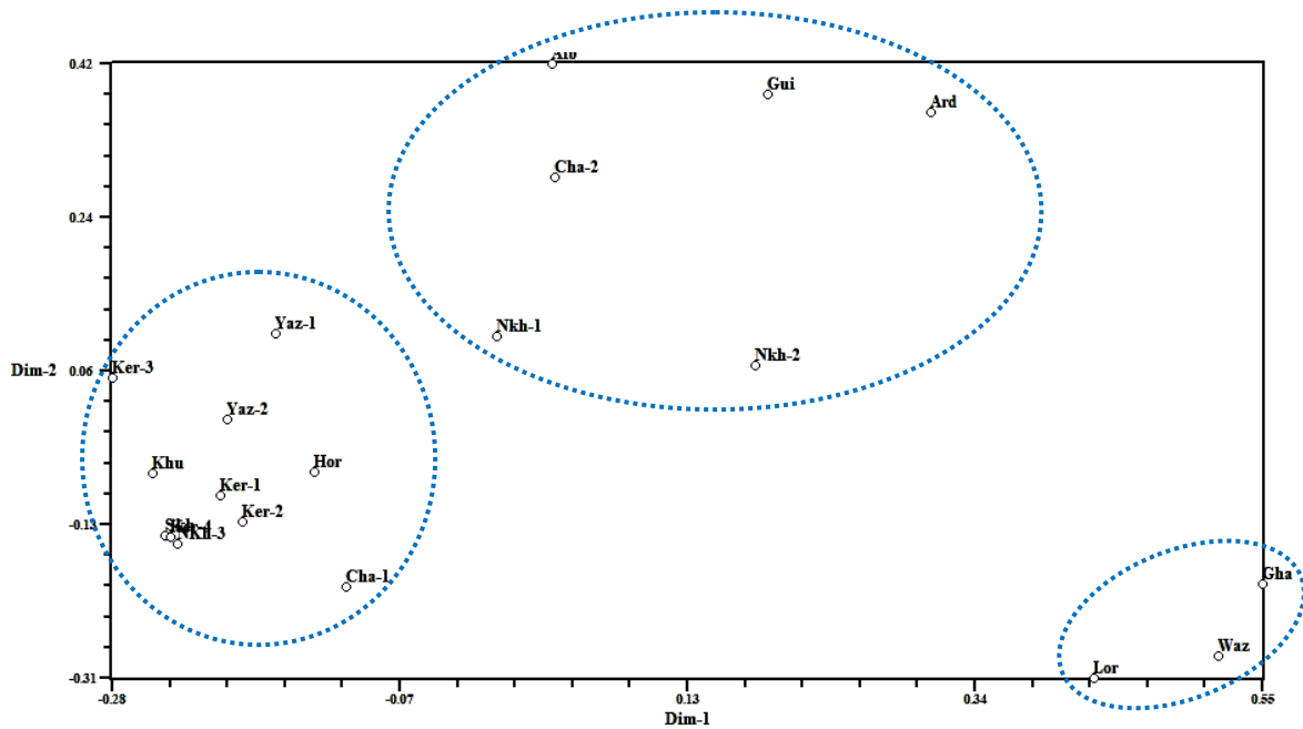
شکل ۳. گروه‌بندی ژنوتیپ‌ها بر اساس تجزیه به مؤلفه‌های هماهنگ اصلی (PCoA)
