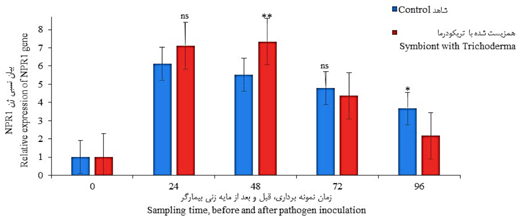
شکل ۳. سطح بیان ژن NPR1 در گیاهان همزیست‌شده با T. harzianum و گیاهان شاهد تلقیح شده با قارچ M. oryzae . ns, ** و * به ترتیب عدم معنی داری؛ معنی دار در سطح احتمال یک درصد و پنج درصد
