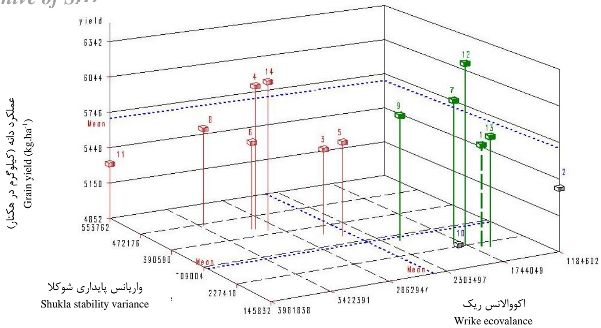
شکل ۲: نمودار سه بعدی پارامترهای واریانس پایداری و اکوالانس در برابر میانگین عملکرد ژنوتیپ‌های برنج Fig. 2: Three-dimensional plot of stability variance and ecovalence stability parameters versus the genotypic mean response in rice genotypes
