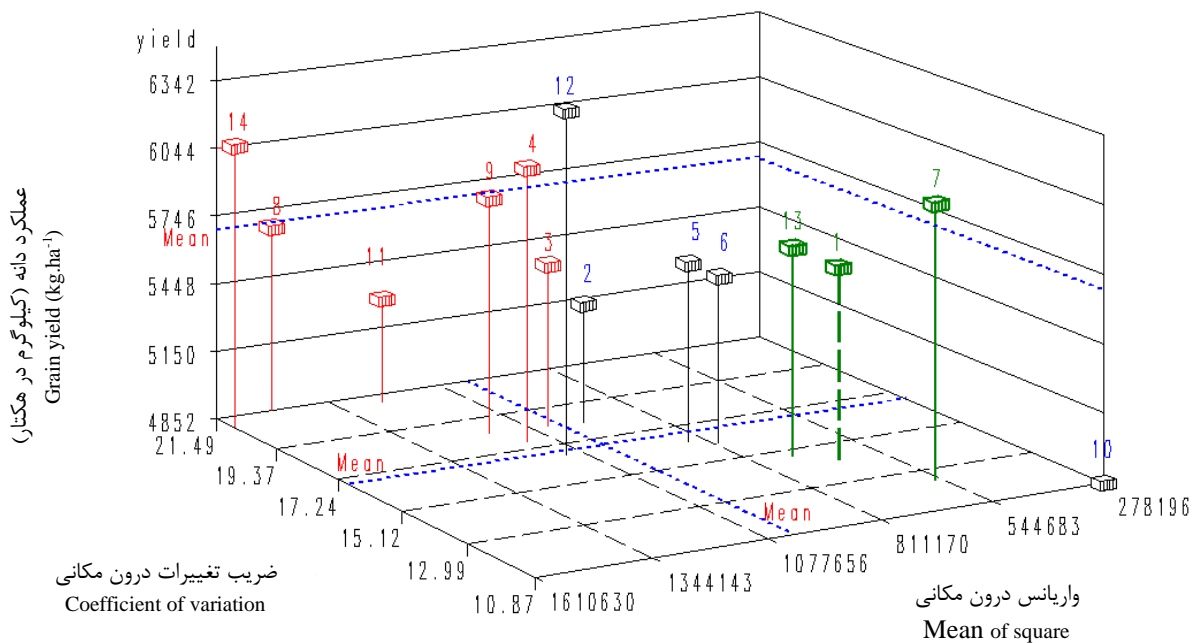
شکل ۳: نمودار سه بعدی پارامترهای واریانس درون مکانی، ضریب تغییرات درون مکانی در برابر میانگین عملکرد ژنوتیپ‌های برنج Fig. 3: Three-dimensional plot of Lin and Binns's stability parameters versus the genotypic mean in rice genotypes
