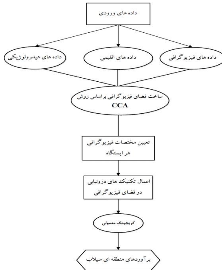
شکل ۲- فلوجارت روش کریجینگ متعارف.
