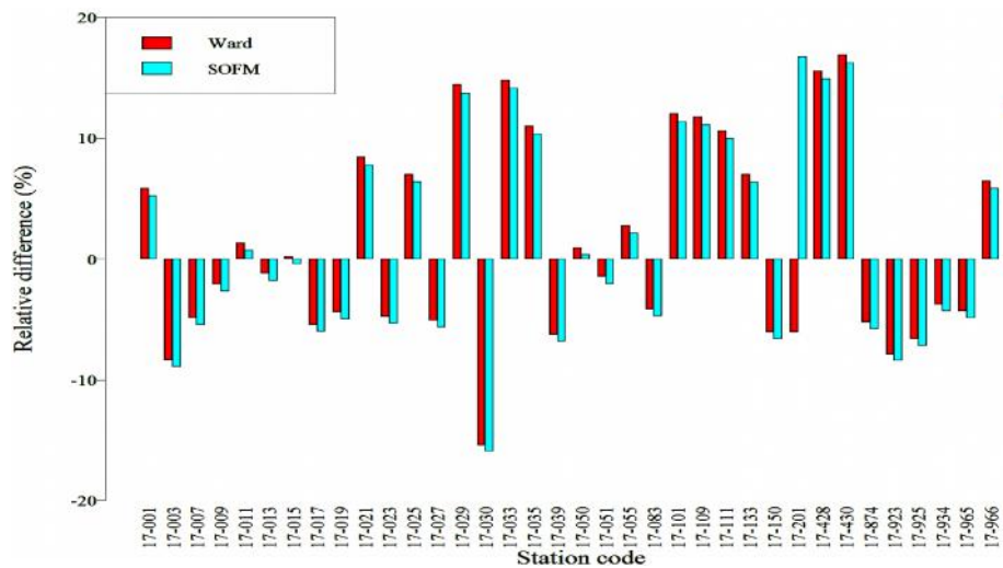
شکل ۱۱- مقایسه‌ی برآوردهای سیلاب با دوره بازگشت ده سال برای ایستگاه‌های مورد مطالعه Figure 11. Comparison of the flood estimates with ten-year return period for the interested stations
