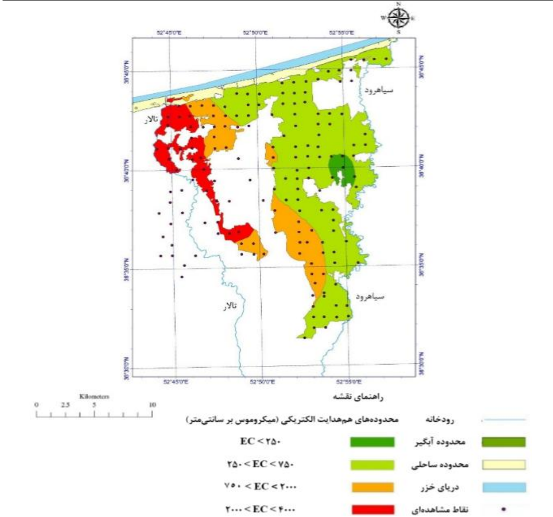
شکل ۴- محدوده‌های با هدایت الکتریکی یکسان در محدوده آبیگر اراضی در پروژه البرز Figure 4. The zones with equal electrical conductivity within Alborz project
