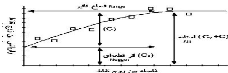
شکل ۳- اجزای مختلف نیم‌تغییرنما (۱۱) Figure 3. The semivariogram components (11)
