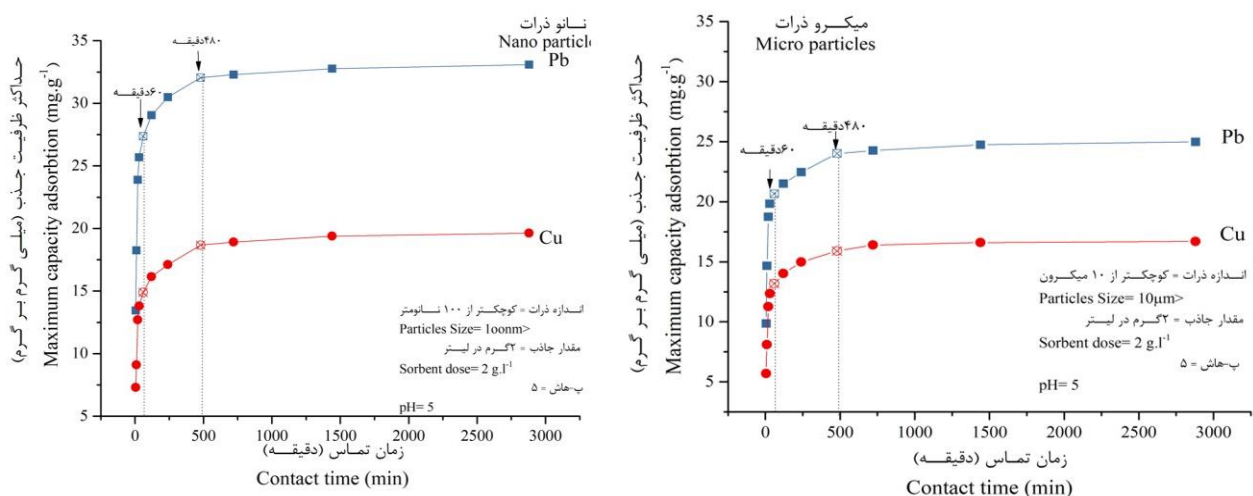
شکل (۳) اثر زمان تماس بر جذب رقابتی سرب و مس از محلول‌های آبی توسط میکرو و نانوذرات پالیگورسکیت
