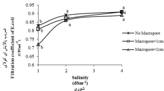
شکل (۳) مقایسه میانگین اثر متقابل قطر ماکروپور و شوری بر ضریب پالایش ای کولای Figure(3) Mean comparison of the interaction between the macrospore diameter and salinity on filtration coefficient of E.coli
