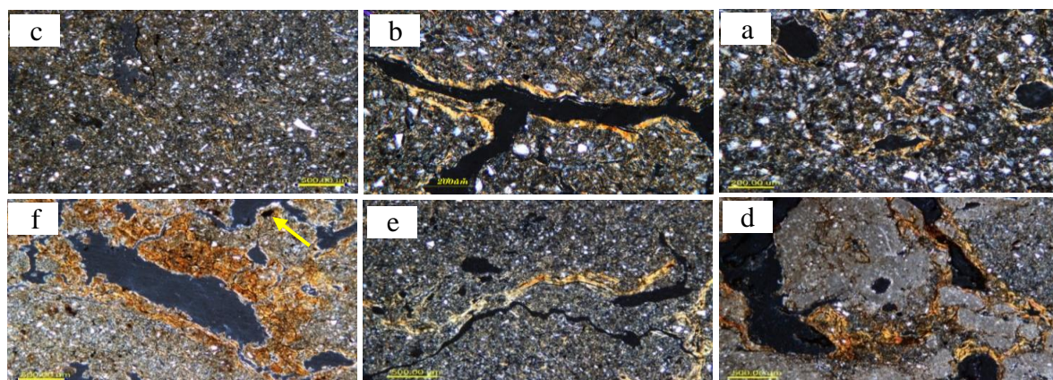
شکل (۳) تصویر مقاطع نازک از پوشش رسی در اطراف حفرات واگ در افق Bt2 قبان (a)، پوشش رسی در داخل کانال در افق Bt2 آق سو (b)، پوشش رسی ضعیف در افق Bt سوسرا (c)، پوشش رسی در اطراف حفره و بی‌فابریک کریستالی در زمینه افق Btk1 توشن (d)، پوشش رسی در اطراف کانال در افق Bt2 النگدره (e)، پوشش رسی پوشیده شده با آهن در اطراف حفره و ندول مگنز که با فلش نشان داده شده است در افق Bt2 نکا (f) (XPL)
