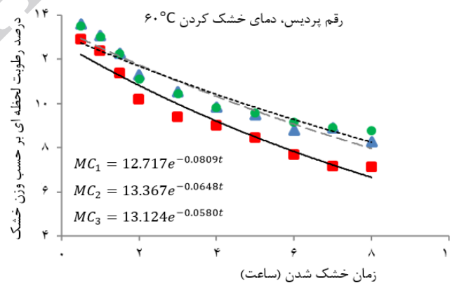
شکل ۴- رابطه زمان و دمای خشک کردن در دمای ۶۰ درجه برای ۴ رقم برنج در سه وضعیت
