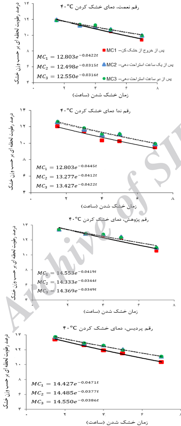
شکل ۲- رابطه زمان و دمای خشک کردن در دمای ۴۰ درجه برای رقم برنج در سه وضعیت
