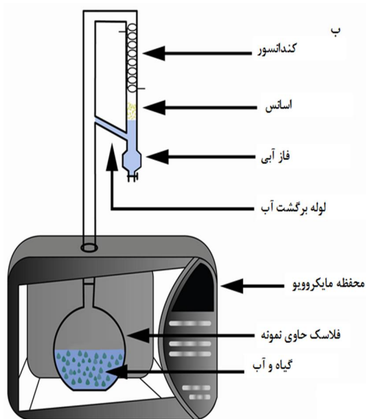
شکل ۱- تجهیزات (الف) تقطیر آبی ساده و (ب) تقطیر آبی به کمک مایکروویو
