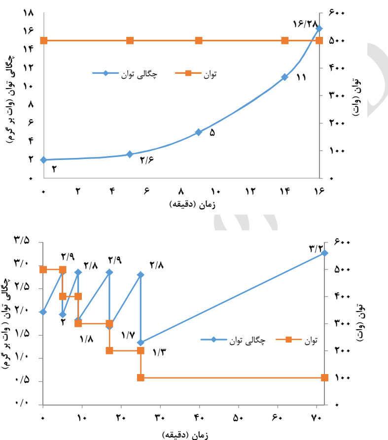
شکل ۲ - تغییرات توان و چگالی توان با زمان (الف) چگالی توان متغیر، (ب) چگالی توان تقریباً ثابت (دمای هوا ۷۰ درجه سلسیوس و چگالی توان ۲ وات بر گرم)
