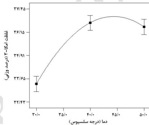
شکل ۴- اثر دما بر درصد تغلیظ امگا-۳ در فشار و سرعت هم‌زدن
