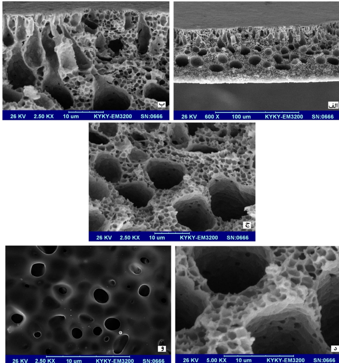
شکل ۲- تصاویر SEM از غشاء پلیمری، (الف) مقطع عرضی کامل؛ (ب) قسمت فوقانی غشاء با حفره‌های ریز؛ (ج) و (د) قسمت تحتانی غشاء با ساختار متخلخل و حفره‌های درشت‌تر؛ (و) سطح غشاء
