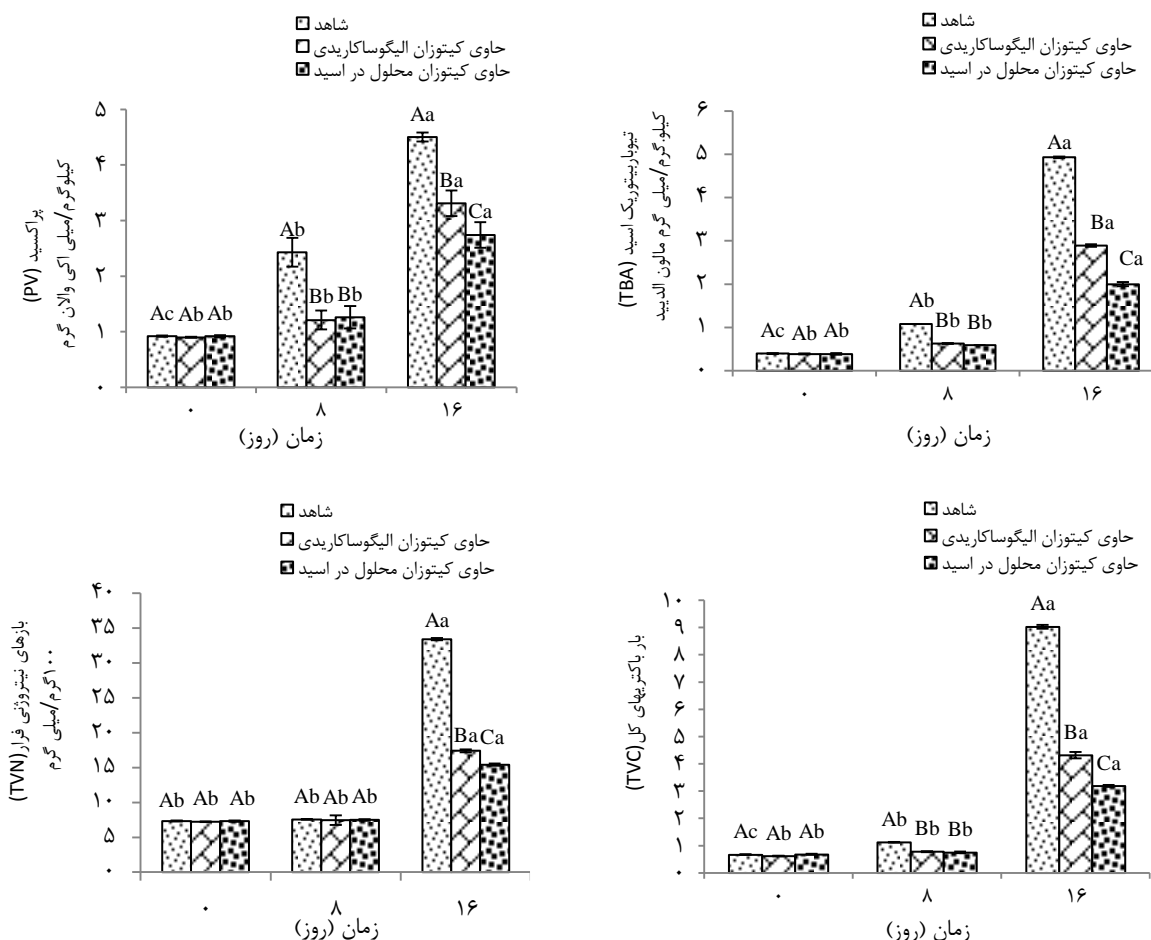
شکل ۲- نتایج حاصل از آنالیز شیمیایی و میکروبی تیمارهای مختلف فیلهٔ فیل ماهی طی نگهداری در یخچال ( 4 \pm 1 درجهٔ سانتی‌گراد) حروف کوچک مقایسهٔ تیمار در زمان، حروف بزرگ مقایسهٔ تیمار به تیمار، نشان‌دهندهٔ اختلاف معنی‌دار در سطح ( P \leq 0.05 ) می‌باشد.
