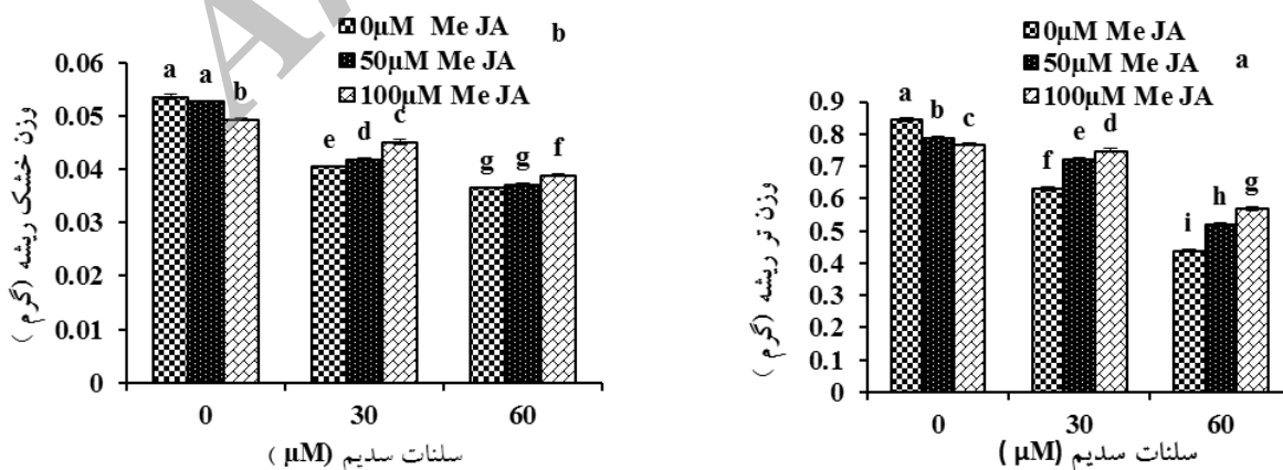
شکل ۳- تاثیر بر هم کنش متیل جاسمونات و سلنات سدیم بر میزان وزن تر (a) و خشک (b) ریشه. کلیه میانگین‌های دارای حداقل یک حرف مشترک از نظر آماری اختلاف معنی‌داری ندارند ( P < 0.001 , mean \pm SE ).
