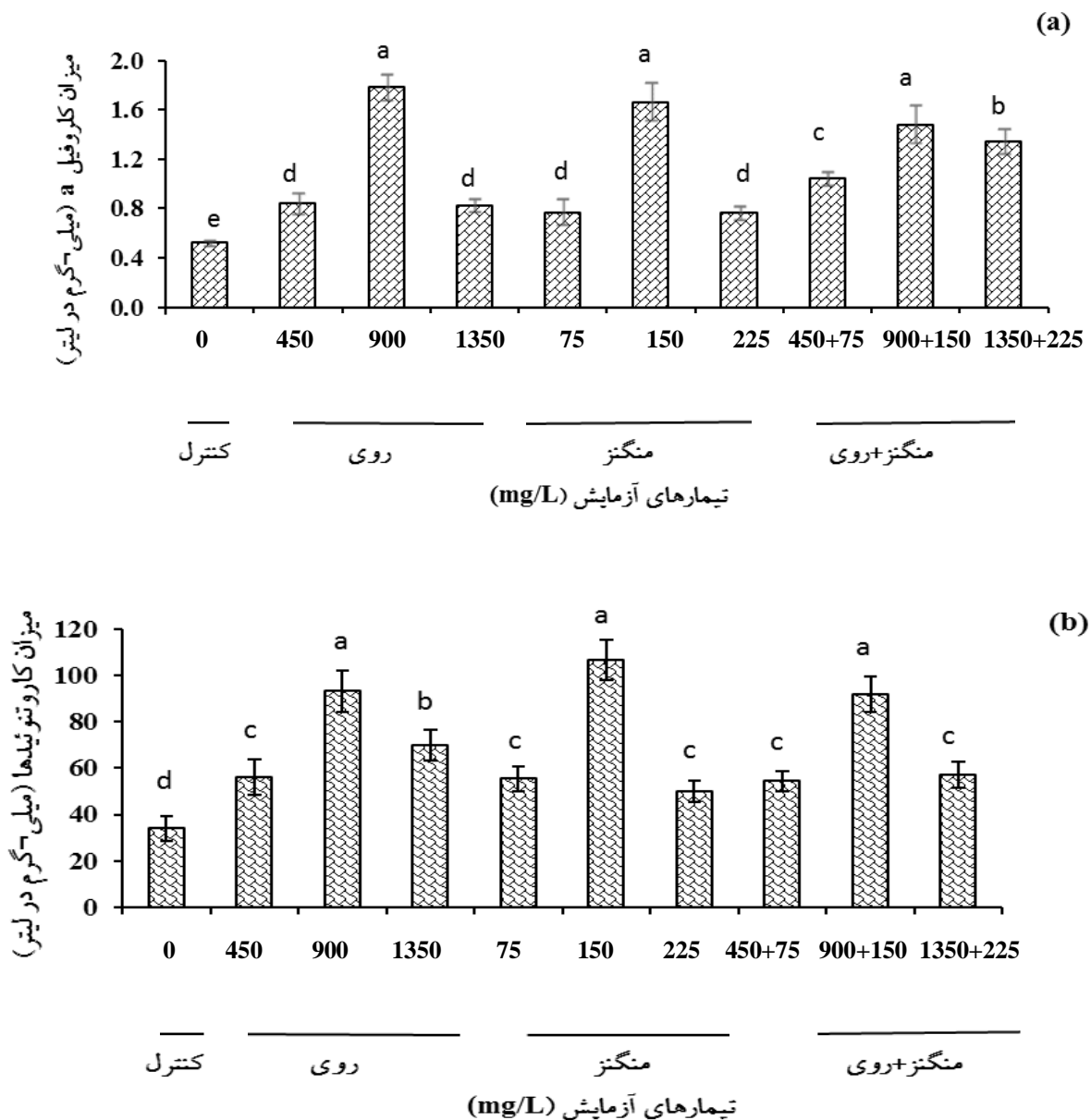
شکل ۳- میانگین (±خطای استاندارد) تأثیرات غلظت‌های مختلف روی، منگنز و ترکیب آنها بر کلروفیل (a) و کل کاروتنوئید (b) در جلبک سبز S. quadricauda . حروف یکسان بیانگر عدم اختلاف معنی‌دار بین میانگین‌ها در سطح ۵ درصد است. اعداد میانگین ۳ تکرار است.
