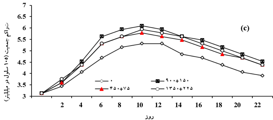
شکل ۱- میانگین تأثیرات غلظت‌های مختلف عنصر روی، منگنز و ترکیب آنها بر پویایی جمعیت در دوره پرورش ۲۲ روزه: (a) روی، (b) منگنز، (c) ترکیب روی و منگنز در جلبک سبز S. quadricauda اعداد میانگین ۳ تکرار است.
