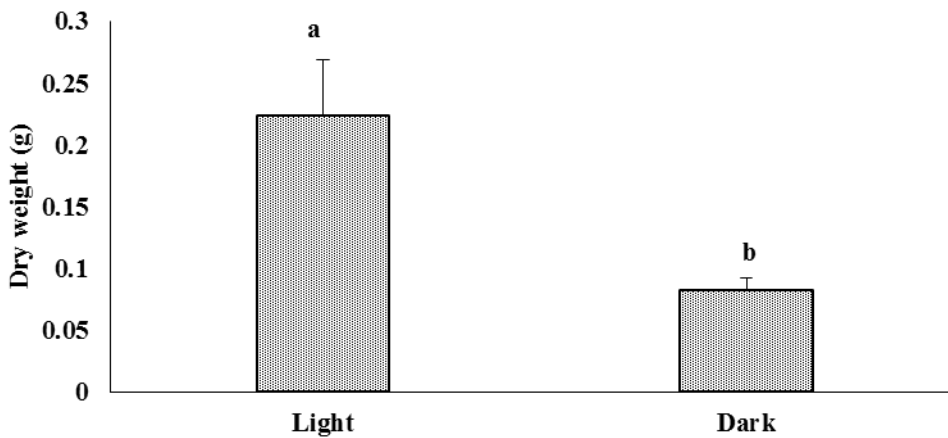
شکل ۲- تاثیر نور بر رشد سلولی در کشت سوسپانسیون سلولی گیاه نوروزک. حروف مشترک بیانگر عدم تفاوت معنی دار است.
