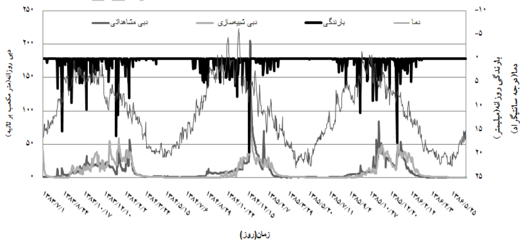
شکل ۵- مقایسه بین دبی مشاهداتی و شبیه‌سازی شده روزانه سال ۸۶-۸۹ برای دوره اعتبارسنجی حوضه دینور
