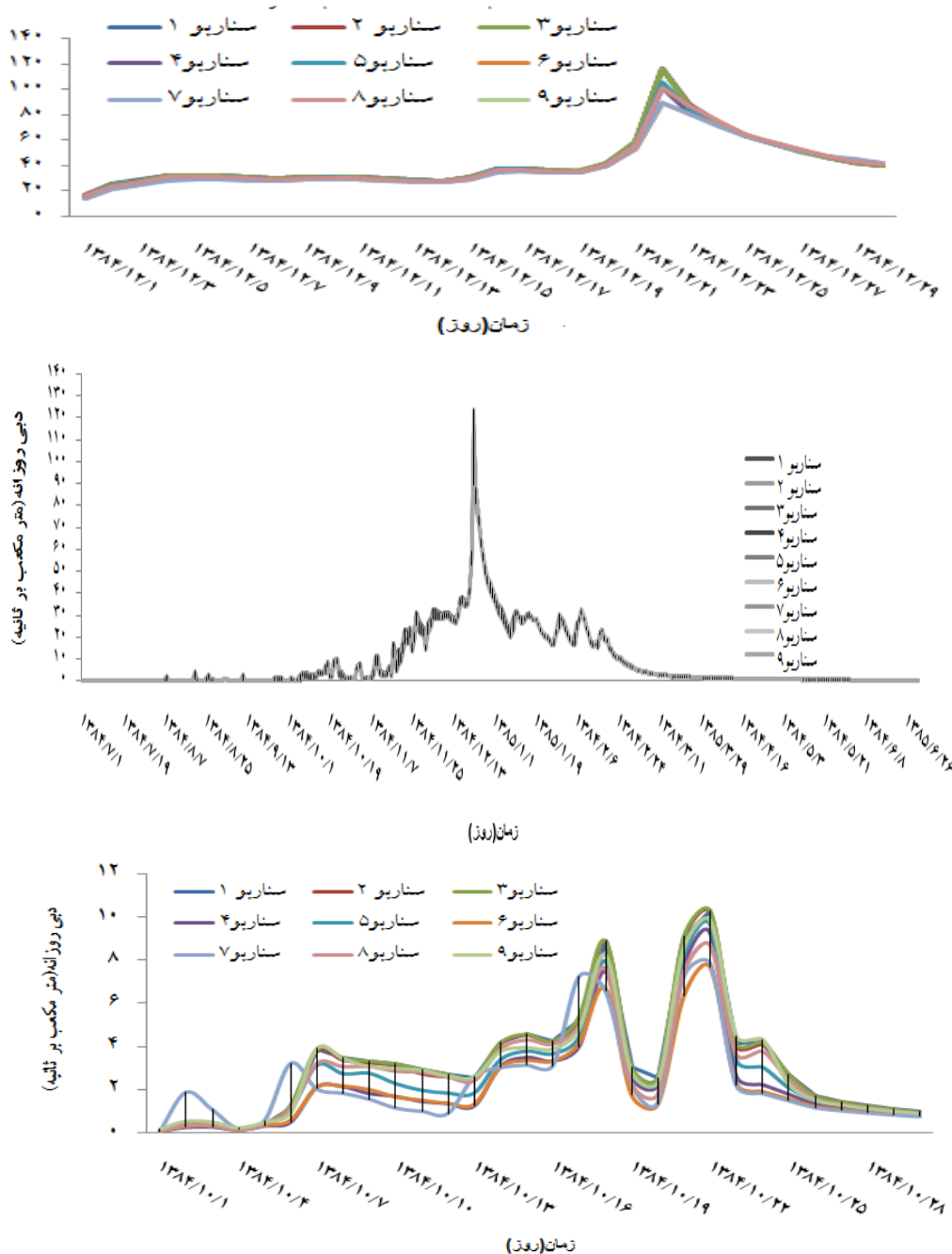
شکل ۷- مقایسه گرافیکی بین دبی شبیه‌سازی شده در سناریو یک (شرایط موجود) و سناریوهای اعمال شده در مدل واسنجی شده در سال آماری ۱۳۸۴-۱۳۸۵
