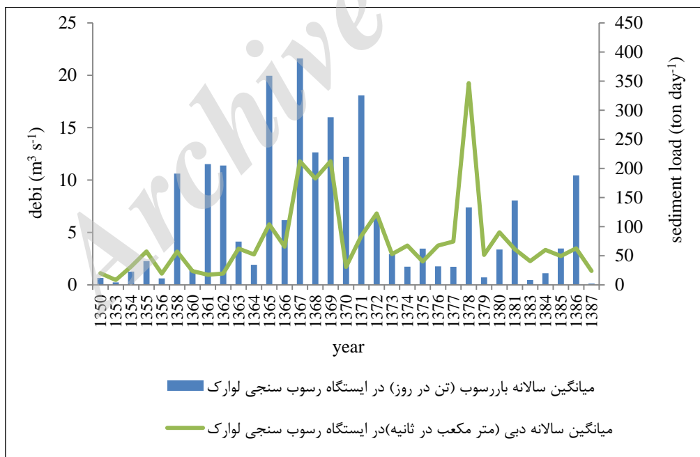
شکل ۳- تغییرات دبی آب و بار رسوب در ایستگاه رسوب‌سنجی علی‌آباد لوارک
