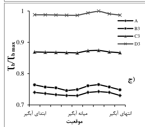
شکل ۱۳- تغییرات تنش برشی بستر در دهانه آبیگر، الف) زاویه نصب آبشکن ۴۵ درجه، ب) زاویه نصب آبشکن ۶۰ درجه، ج) زاویه نصب آبشکن ۹۰ درجه و د) آزمایش‌های نوع C
