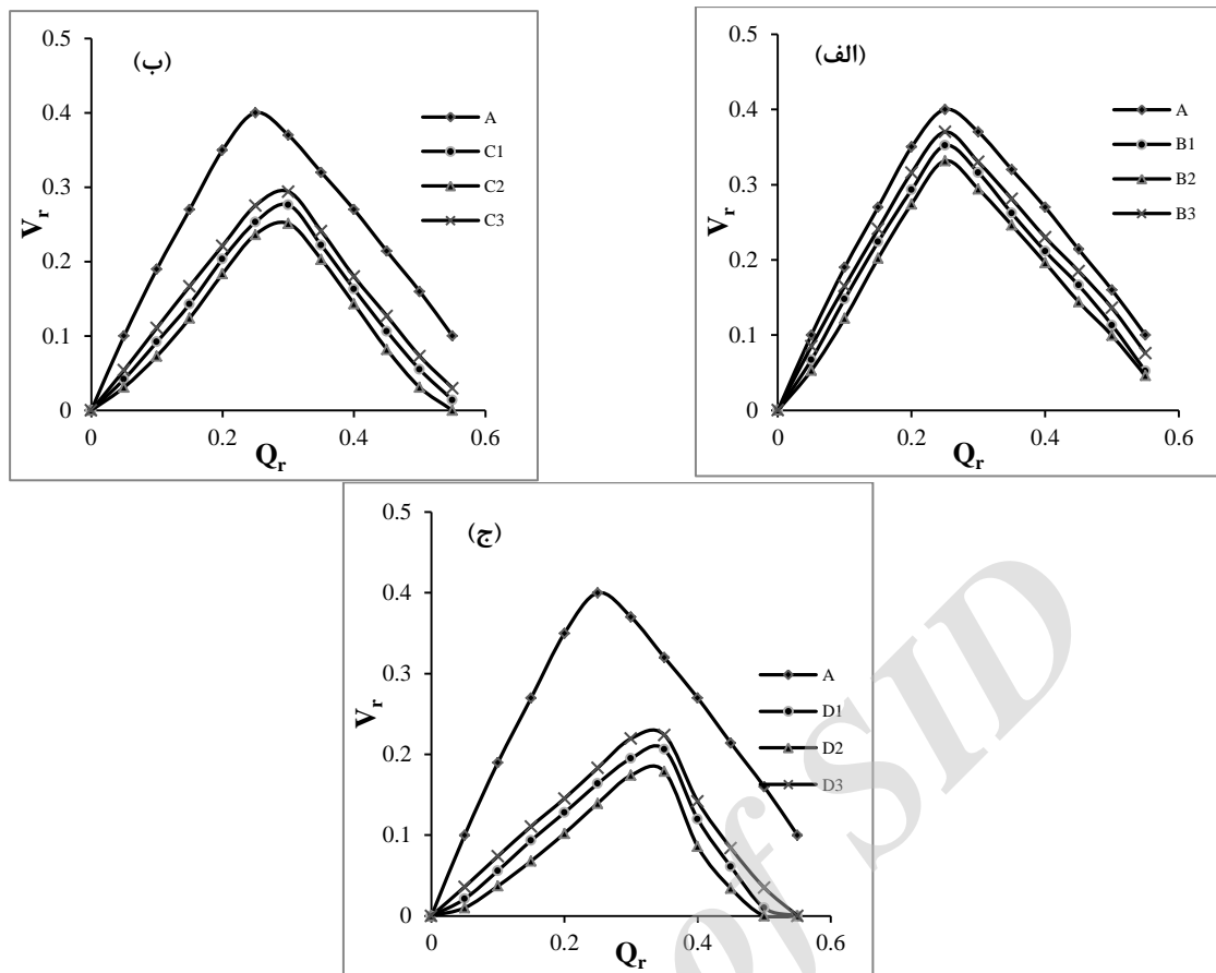
شکل ۸- تغییرات نسبت حجم رسوب ته‌نشین شده در برابر نسبت آبگیری، الف) آزمایش‌های نوع B، ب) آزمایش‌های نوع C و ج) آزمایش‌های نوع D
