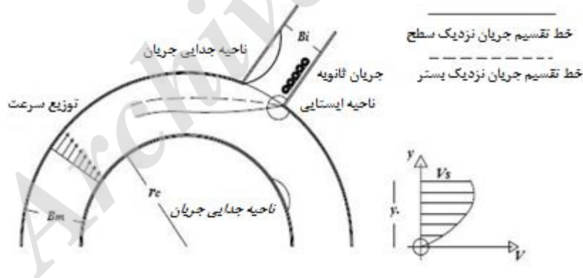
شکل ۱- ویژگی‌های جریان انحرافی به آبنگیز در کانال‌های باز
