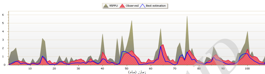
شکل ۸- نتایج حاصل از اجرای مدل در مرحله واسنجی برای شبیه‌سازی رواناب در ایستگاه کارخانه سیمان
