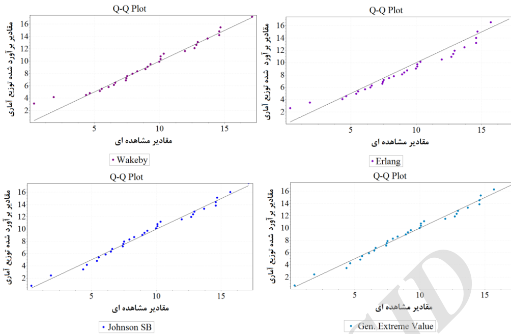
شکل ۶- نمودارهای Q-Q با مدت دوام یک روزه رودخانه شهرچای
