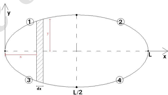
شکل ۱- شماتیکی از هندسه حوزه آبخیز در نظر گرفته شده در مدل زمان-مساحت
