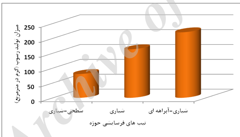
شکل ۵- نمودار مقایسه میانگین رسوب تولیدی در تیپ‌های مختلف فرسایشی حوضه
