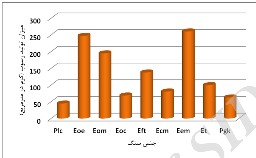
شکل ۴- نمودار مقایسه میانگین تولید رسوب در سنگ‌های مختلف حوضه
