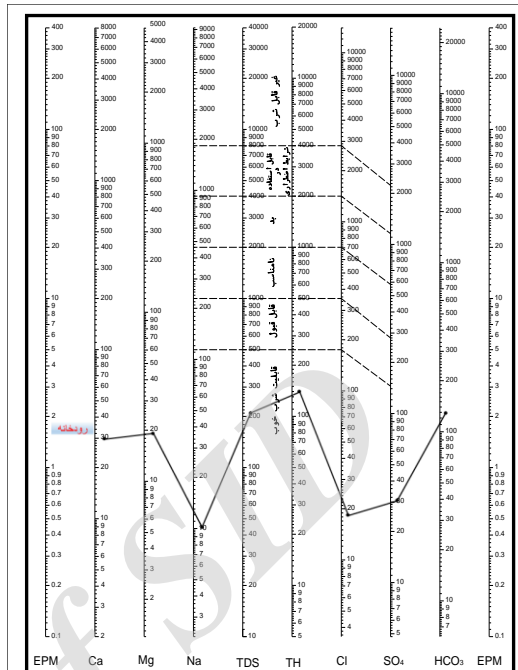
شکل ۱۰- الف) دیاگرام شولر دوره خشک سال ۱۳۹۲، ب) دیاگرام شولر دوره مرطوب سال ۱۳۹۲
