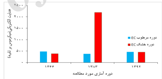
شکل ۱۱- متوسط هدایت الکتریکی دوره مرطوب و خشک زرينه‌رود
