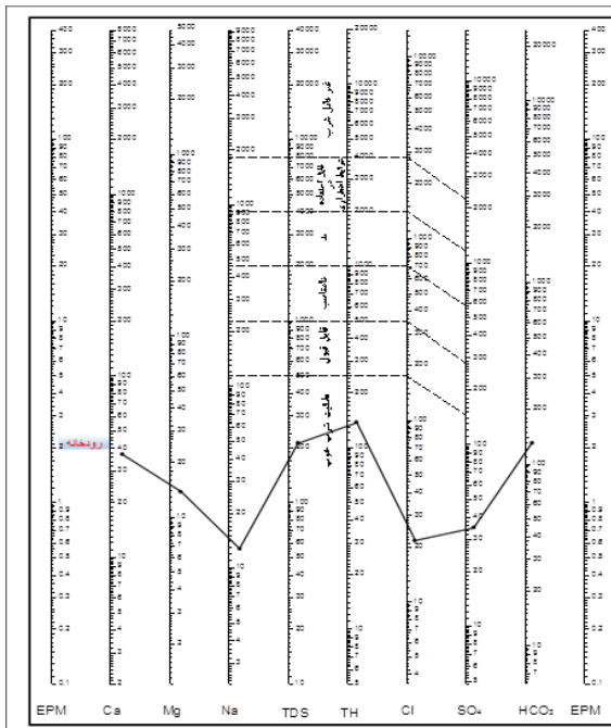
شکل ۱۰- الف) دیاگرام شولر دوره خشک سال ۱۳۹۲، ب) دیاگرام شولر دوره مرطوب سال ۱۳۹۲
