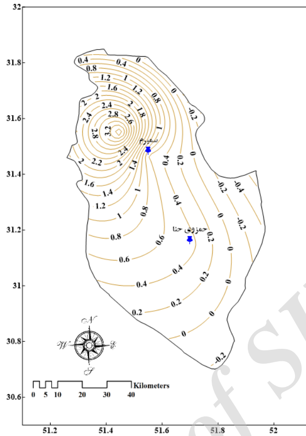
شکل ۲- نقشه خطوط هم‌روند میانگین دمای سالانه در منطقه سمیرم
