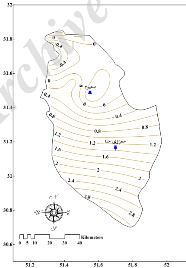
شکل ۳- نقشه خطوط هم‌روند میانگین دمای بیشینه سالانه در منطقه سمیرم
