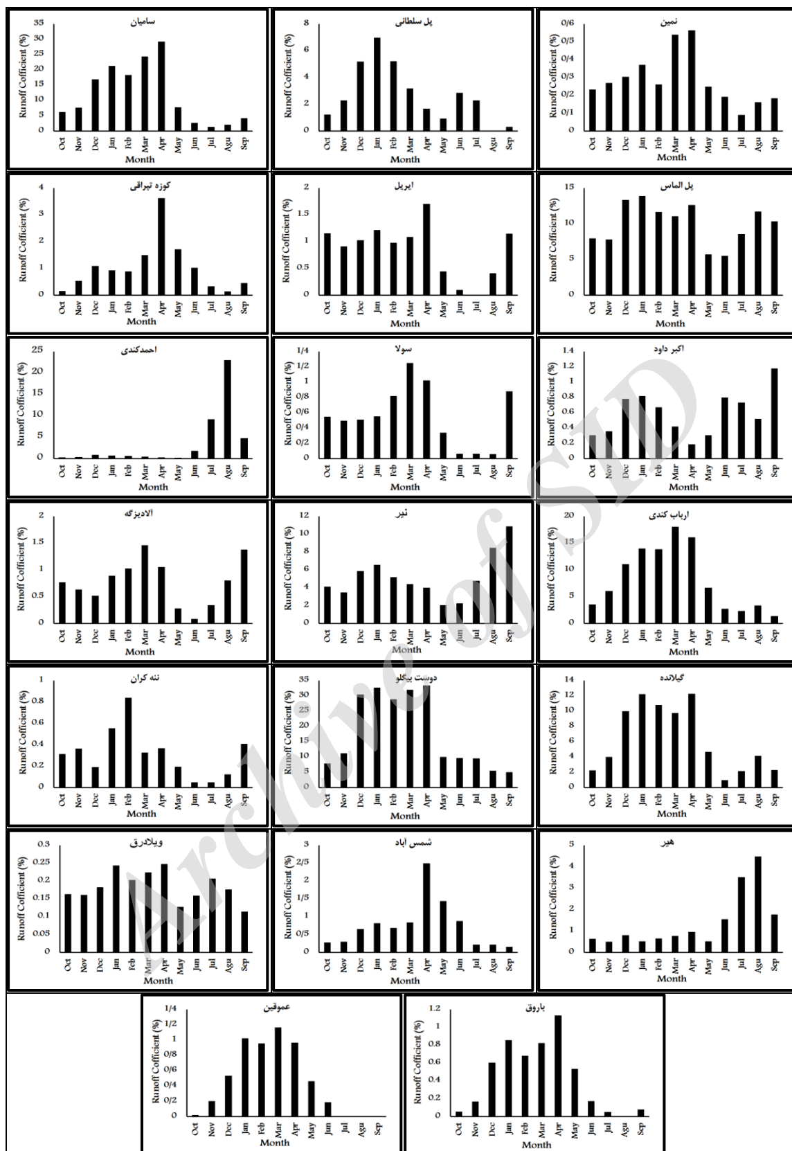
شکل ۳- توزیع زمانی مقادیر ضریب رواناب در ماه‌های مختلف در حوضه‌های استان اردبیل
