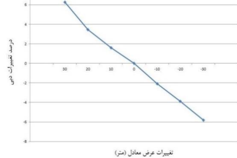
شکل ۱۱- تغییرات عرض معادل و تأثیر آن بر دبی اوج
