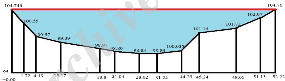
شکل ۸- نمای شماتیک از مقطع اندازه‌گیری شده
