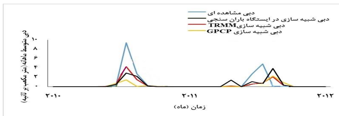
شکل ۶- هیدروگراف دبی مشاهده‌ای و شبیه‌سازی شده در دوره صحت‌سنجی
