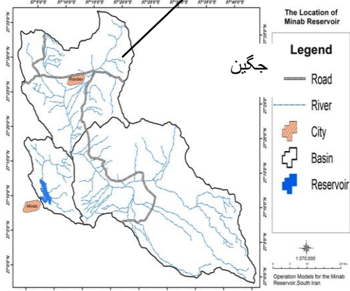
شکل ۱- موقعیت مخزن و زیرحوضه‌های منطقه میناب در استان هرمزگان (Army Geographic Agency, ۲۰۰۷)
