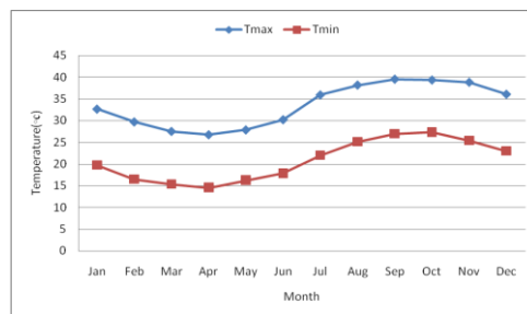
شکل ۶- متوسط بیشینه و کمینه درجه حرارت ماهانه در ایستگاه میناب (Hormozgan Province Meteorological Organization, ۲۰۰۷)
