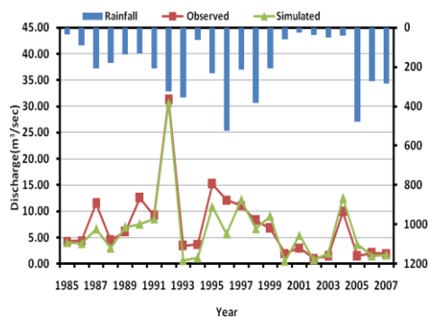
شکل ۱۰- آبدهی مشاهده‌ای و برآورد شده سالانه میناب
