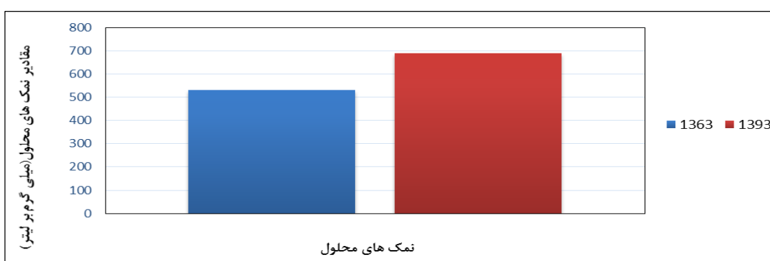
شکل ۱۴- تغییرات نمک‌های محلول در رودخانه شاوور سال ۱۳۶۳-۱۳۹۳
