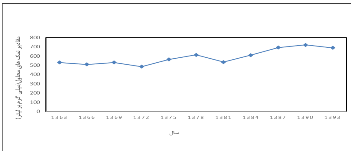
شکل ۱۳- روند تغییرات TDS در رودخانه شاوور سال ۱۳۶۳-۱۳۹۳
