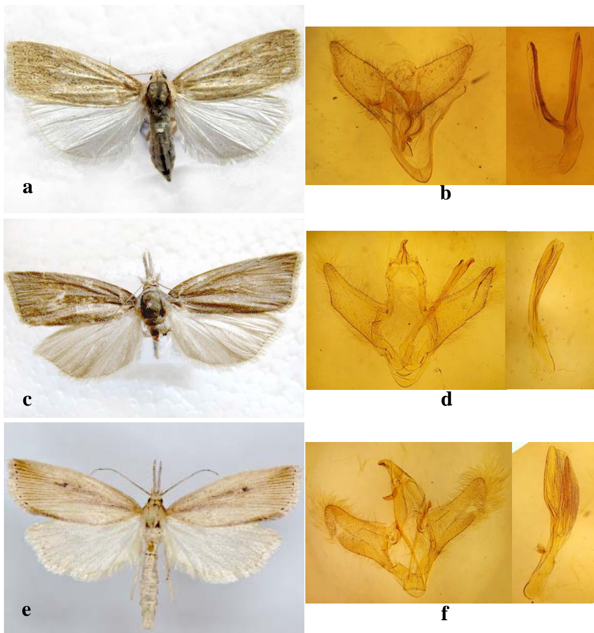
شکل ۲- (a) حشره‌ی بالغ ماده Chilo suppressalis ; (b) اندام تولیدمثلی خارجی نر Chilo suppressalis ; (c) حشره‌ی بالغ ماده C. suppressalis ; (d) اندام تولیدمثلی خارجی نر Chilo luteellus ; (e) حشره‌ی بالغ ماده Chilo phragmitella ; (f) اندام تولیدمثلی خارجی نر C. phragmitella
