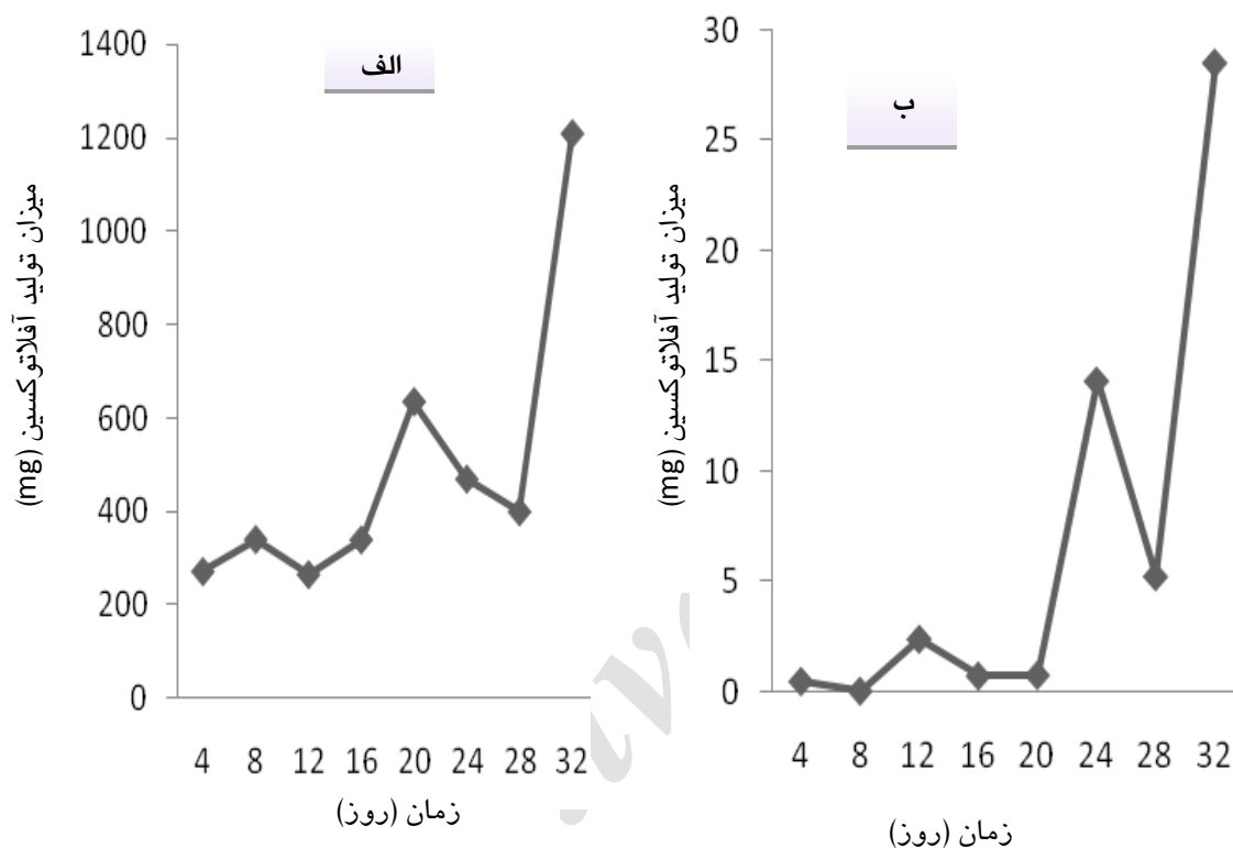
شکل ۲- میزان تولید آفلاتوکسین طی ۳۲ روز در A. flavus (الف) و A. foetidus (ب) بر حسب میلی‌گرم در ۵۰ میلی‌لیتر محیط PDB.
